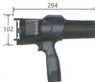
尺寸 (mm)
